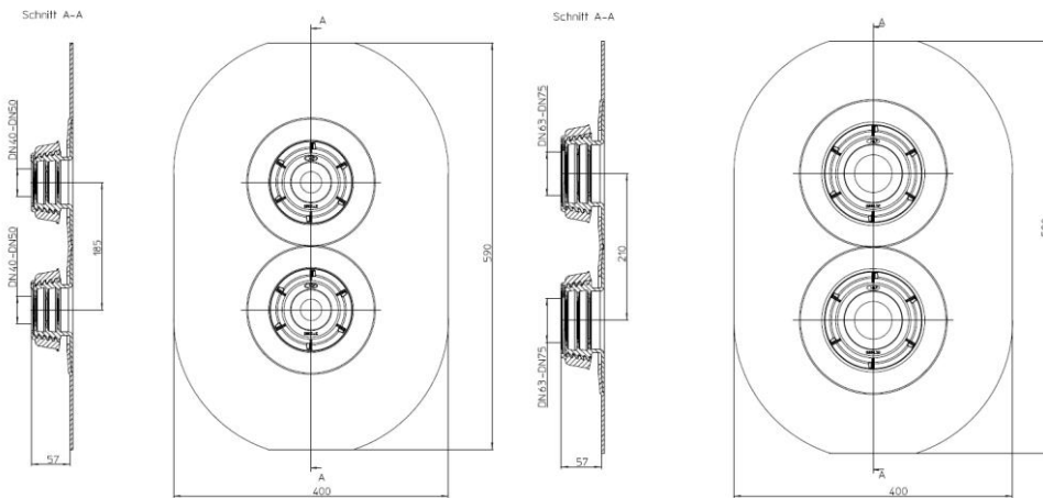
Рис. 1. HL800.2/40-50
