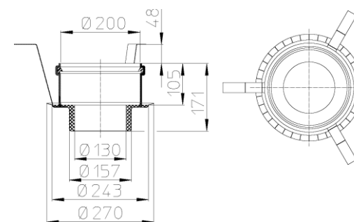
Рис. 2. Противопожарная муфта HL860 для трапа HL616HLW/1.
