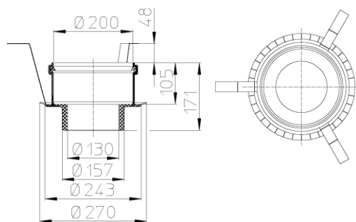
Рис. 2. Противопожарная муфта HL860 для трапа HL616W/1.
