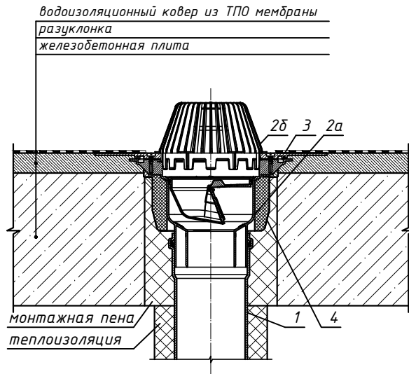
2. Трап HL3100Т.3
