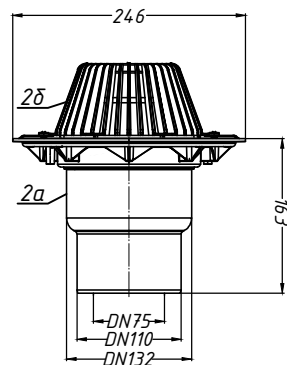
2. Трап HL3100Т.3
