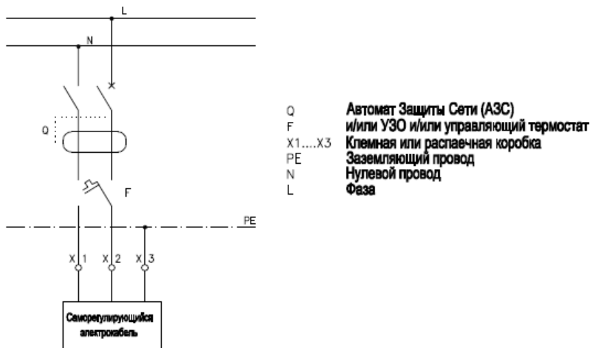
Рис. 1. Электрическая схема подключения кабеля электрообогрева.
