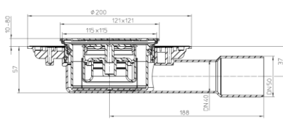
Рис. 2. Трап HL90.Prblue-3000
