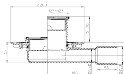
Рис. 3. Трап HL90
