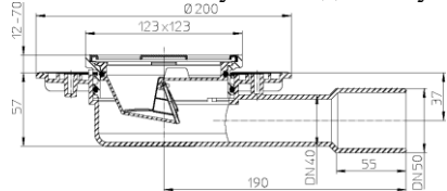
Рис. 1. Трап HL90.2
