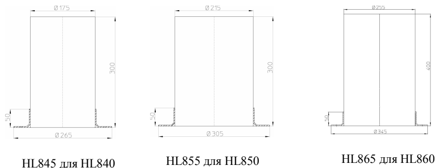
Рис. 2. Закладные элементы для противопожарных муфт.
