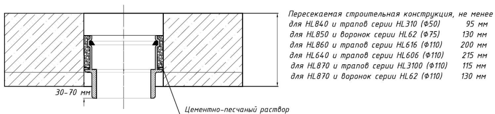
Рис.3. Схема установки противопожарной муфты.
