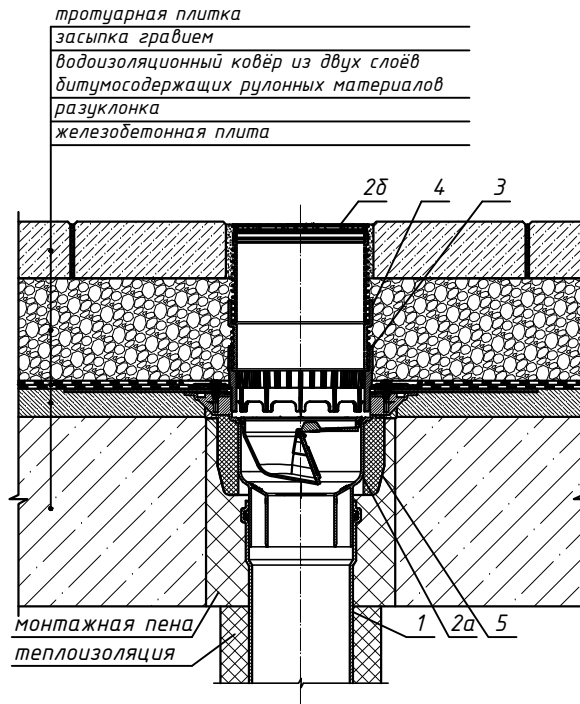
2. Трап HL3100TH
