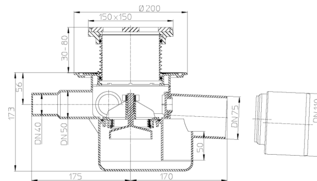
Рис.1. Трап HL70G
