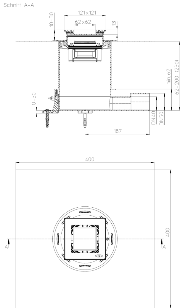
Рис. 2. Трап HL541I.
