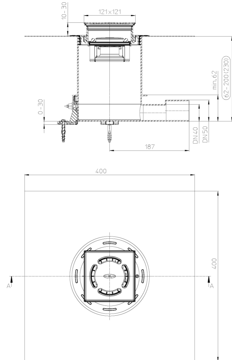
Рис. 1. Трап HL541.
