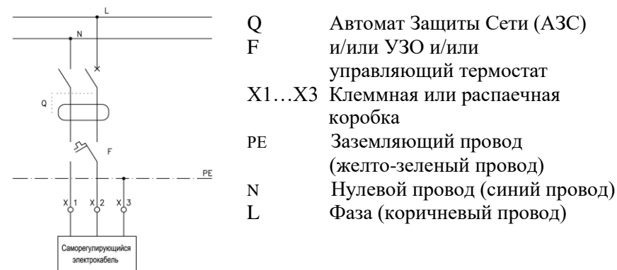
Рис. 3. Схема подключения электрообогрева кровельной воронки HL64.1BF к электрической сети.
