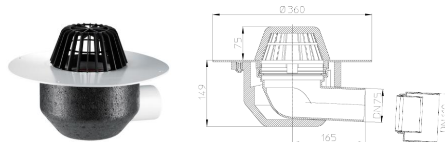
Рис. 1. Кровельная воронка HL64P.
