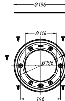
4. Обжимной фланец HL83.0
