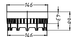
6. Дренажное кольцо HL150
