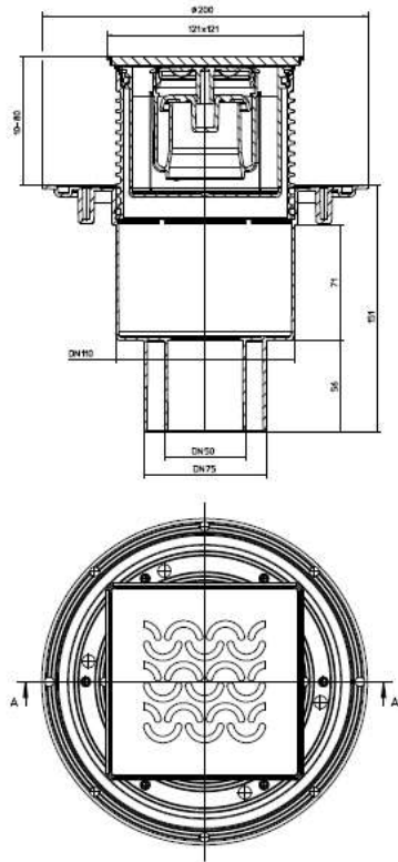
Рис. 1. Трап HL310Prblue-3121
