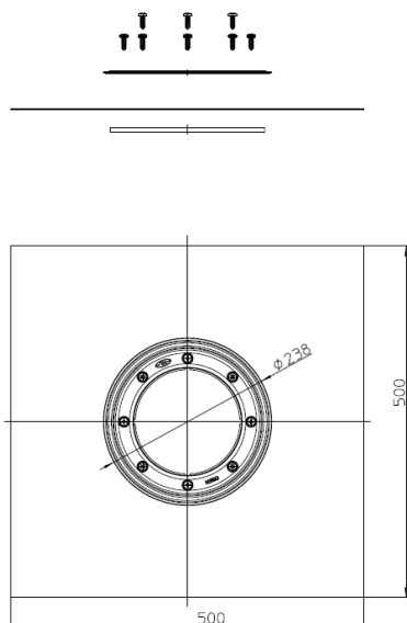
Рис.1. Гидроизоляционный фланец HL8300.
