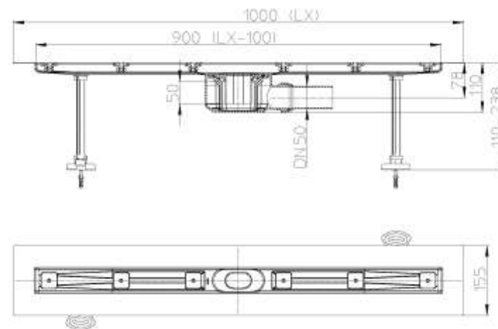
Рис. 1. Корпус лотка HL50F.0/100.
