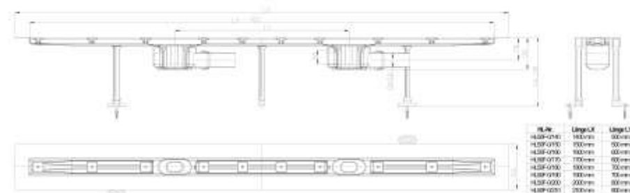
Рис. 2. Корпус лотка с двумя сифонами.
