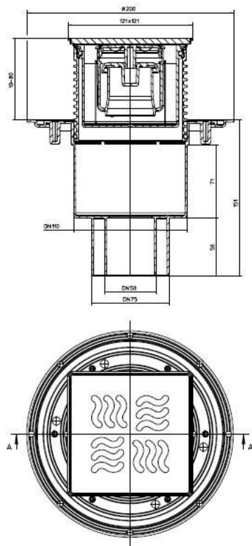
Рис. 1. Трап HL310Prblue-3125.
