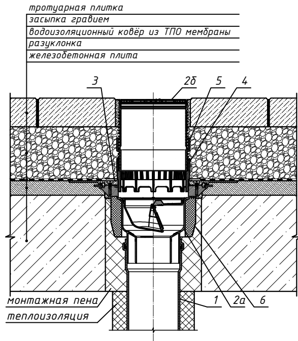
2. Трап HL3100T
