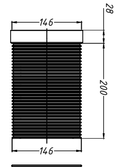
5. Удлинитель HL3400
