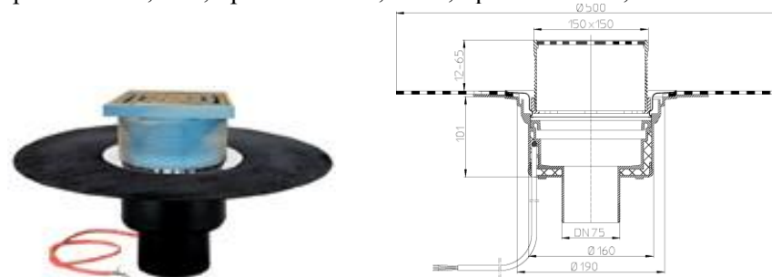
Рис. 1. Кровельная воронка с электрообогревом HL62.1BH/7.
