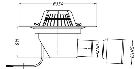
3. Воронка HL64.1
