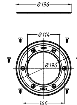
4. Обжимной фланец HL83.0
